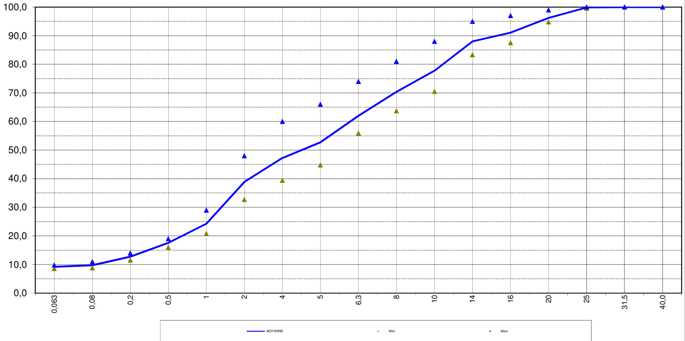
Analyse granulometrique par tamisage selon la norme NF EN 933-1
